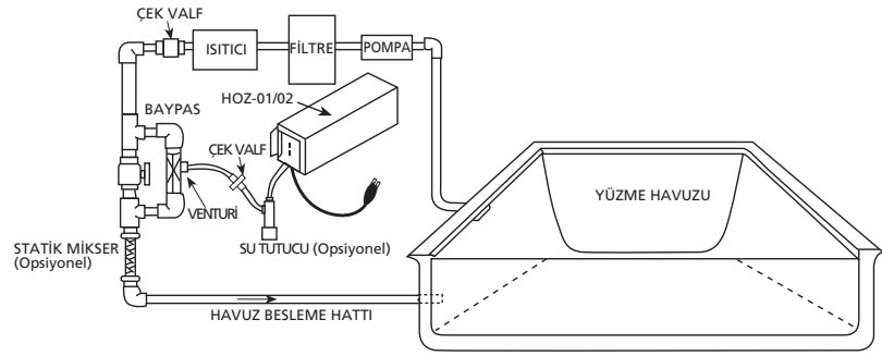
MONTAJ ŞEMASI
