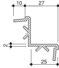
PVC Profil. Üstten taşma Membranlı Havuzlar için özel Kanal Kenar Profili
