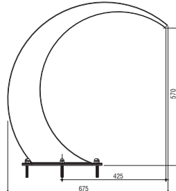
Yandan görünüş
