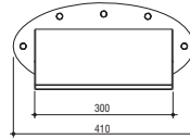
Önden görünüş
