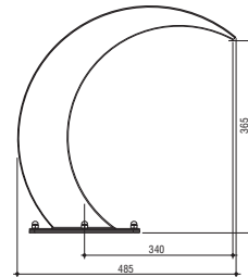
Yandan görünüş
