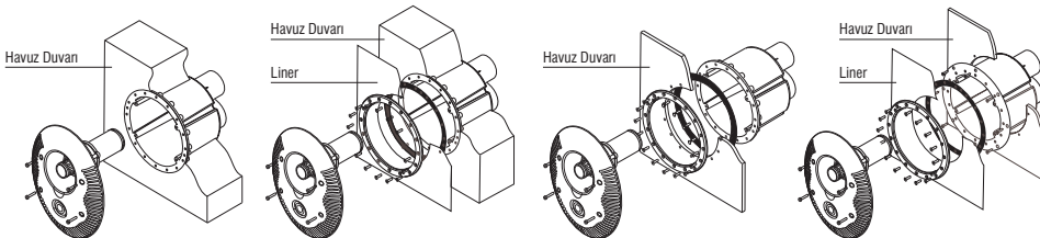
Beton Yüzme Havuzu
