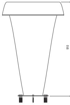
Önden görünüş
