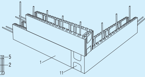
Şekil 3: Stropor bloğun köşe dönüşlerde dönüş birleşimi
