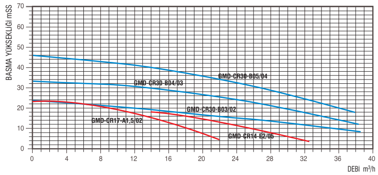
PERFORMANS EĞRİLERİ
